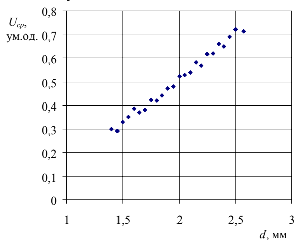
Рисунок 5 – Експериментально отримана залежність вихідного сигналу магнітоелектричної системи від середньозваженої крупності пісового матеріалу
