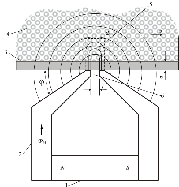
Рисунок 2. Магнітна система з постійними магнітами:
