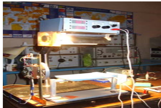
Рисунок 1. Експериментальна установка, загальний вид
