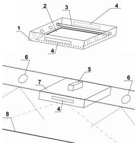
Рисунок 5. Пристрій аварійного освітлення
